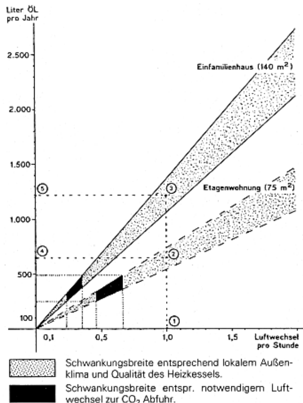
Abb. 2: Heizenergieverbrauch für die Lüftung in Abhängigkeit von der durchschnittlichen Luftwechselrate.
