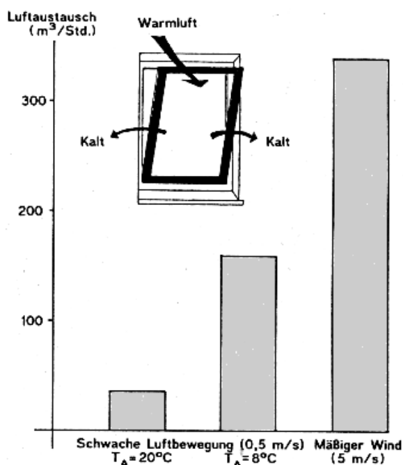
Abb. 9: Luftaustausch an einem gekippten Fenster durch Thermik und Windeinfluss.
