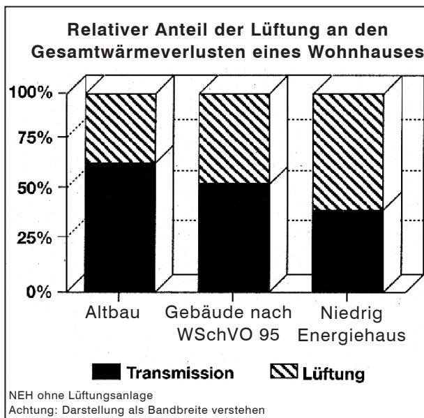
Abb. 1: Relativer Anteil der Lüftung an den Gesamtwärmeverlusten eines Wohnhauses
