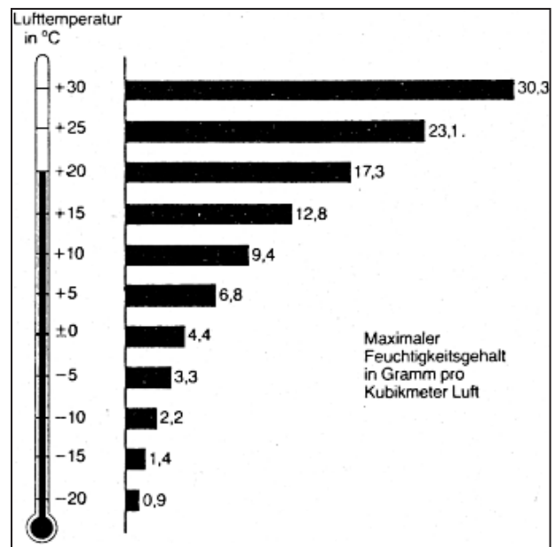
Abb. 5: Maximaler Wasserdampfgehalt (= 100 % relative Luftfeuchte) in Gramm pro m 3 Luft bei verschiedenen Temperaturen.
