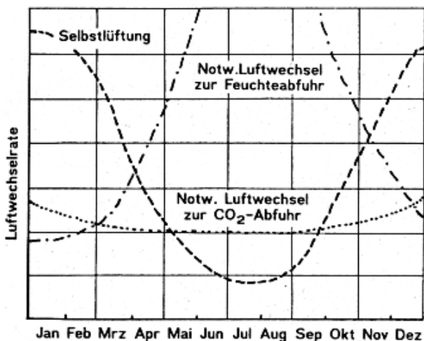
Abb. 7: Qualitativer, jahreszeitlicher Verlauf der Selbstlüftung bei Fenstern ohne Fugendichtung im Vergleich mit der notwendigen Luftwechselrate (ohne Berücksichtigung des Windeinflusses).
