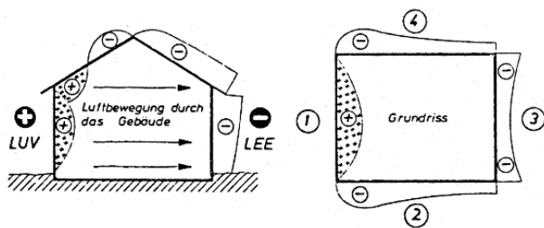
Abb. 10: Winddruck und -sog bei einem freistehenden Gebäude
