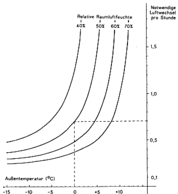
Abb. 6: Notwendige Luftwechselraten zur Wasserdampfabfuhr in Abhängigkeit von der Außentemperatur. (Rahmendaten: Relative Luftfeuchtigkeit außen = 100 %, Wasserdampfproduktion in der Wohnung 500 g/Stunde, Etagenwohnung 75 m 2 ).
